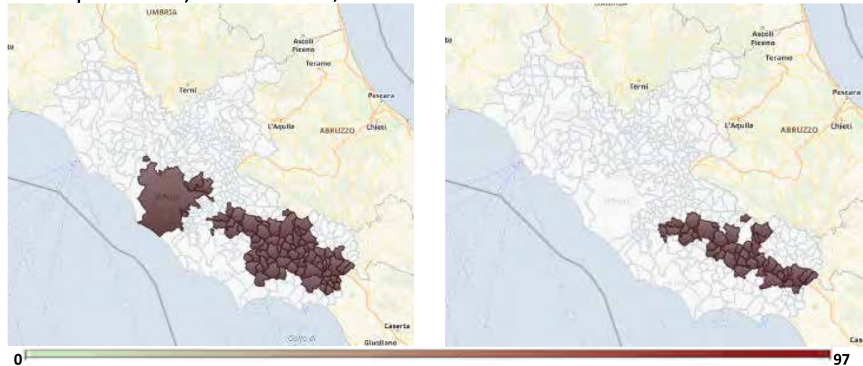
Grafico 1.16: Particolato inferiore a 10 micron, numero di superamenti del valore soglia limite giornaliero di 50 µg/m3 (numero superamenti=35) - Lazio - Anni 2013, 2023
