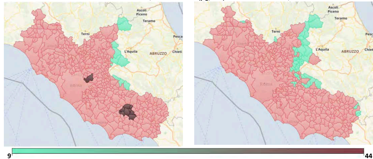
Grafico 1.14: Particolato inferiore a 10 micron, media annua (µg/m3) – Lazio - Anni 2013, 2023
