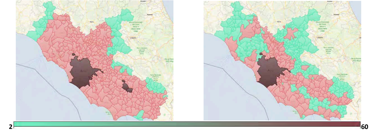
Grafico 1.20: Biossido di azoto (NO2) - media annua (µg/m3, valore soglia 40 µg/m3); Lazio - Anni 2013, 2023
