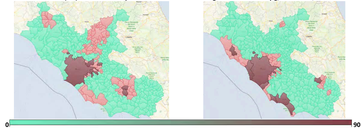
Grafico 1.22: Ozono (O3) - numero di superamenti del valore limite giornaliero di 120 µg/m3 - Lazio, 2013 vs 2023
